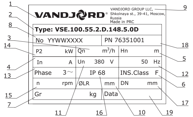
Рис. 2 Фирменная табличка
