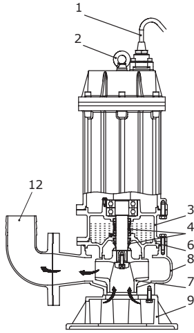
Рис. 1 Насос VS, VSE
